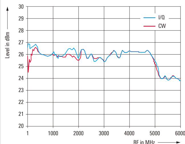
测得的最大输出功率/频率图
