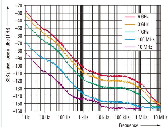
使用内部的OCXO测得的SSB相位噪声
