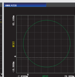
导纳圆图显示画面
