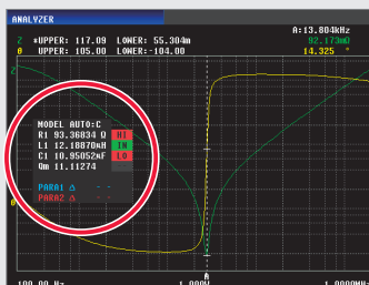
对等效电路各元件进行合格与否判定的画面
