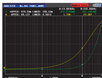
频率扫描测量 Z-θ 测量画面
