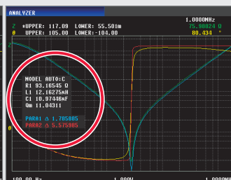
分析结果模拟画面
