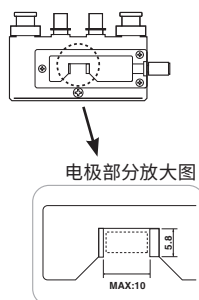
SMD 测试治具 9263
