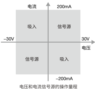
源动作(高精度电源)
