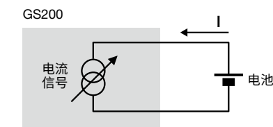
吸入动作(高精度负载)
