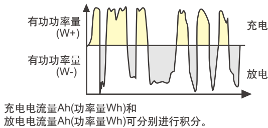
典型的重复性高速充电和放电信号
