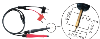
9770前端形状
