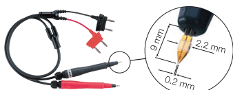
9771前端形状
