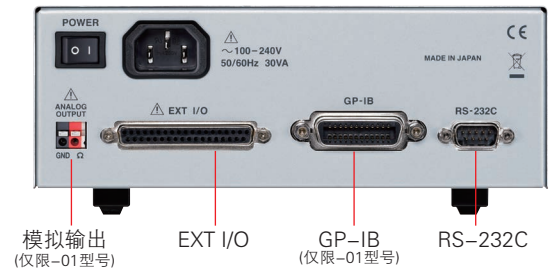
BT356-01、BT3562-01 背面
