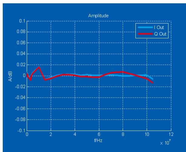
最高 100 MHz/Q 带宽时，典型值为 0.05 dB 的高线性频率响应
